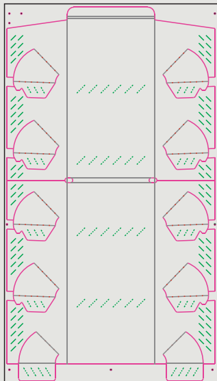
Corpo Papelão EB 4/4 - 89x158cm x6700
