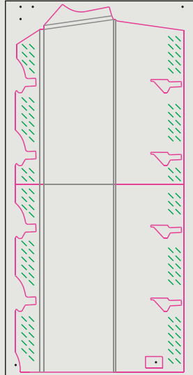
Lateral esquerda Papelão EB 4/0 - 77x153cm x6700
