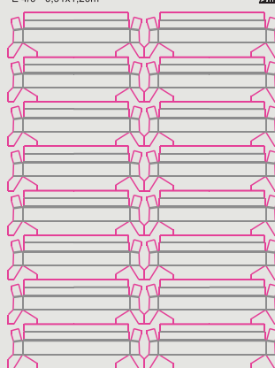
Frente de prateleira E 4/0 - 0,91x1,20m
