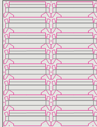
Frente de prateleira Papelão E 4/0 - 93x122cm x1675
